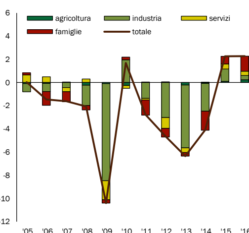
FIGURA II.23: CONTRIBUTO SETTORIALE ALLA VARIAZIONE DELLE EMISSIONI TOTALI DI CO2 - ANNI 2005-2016(*)
